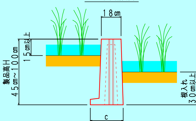
ブロック断面図
